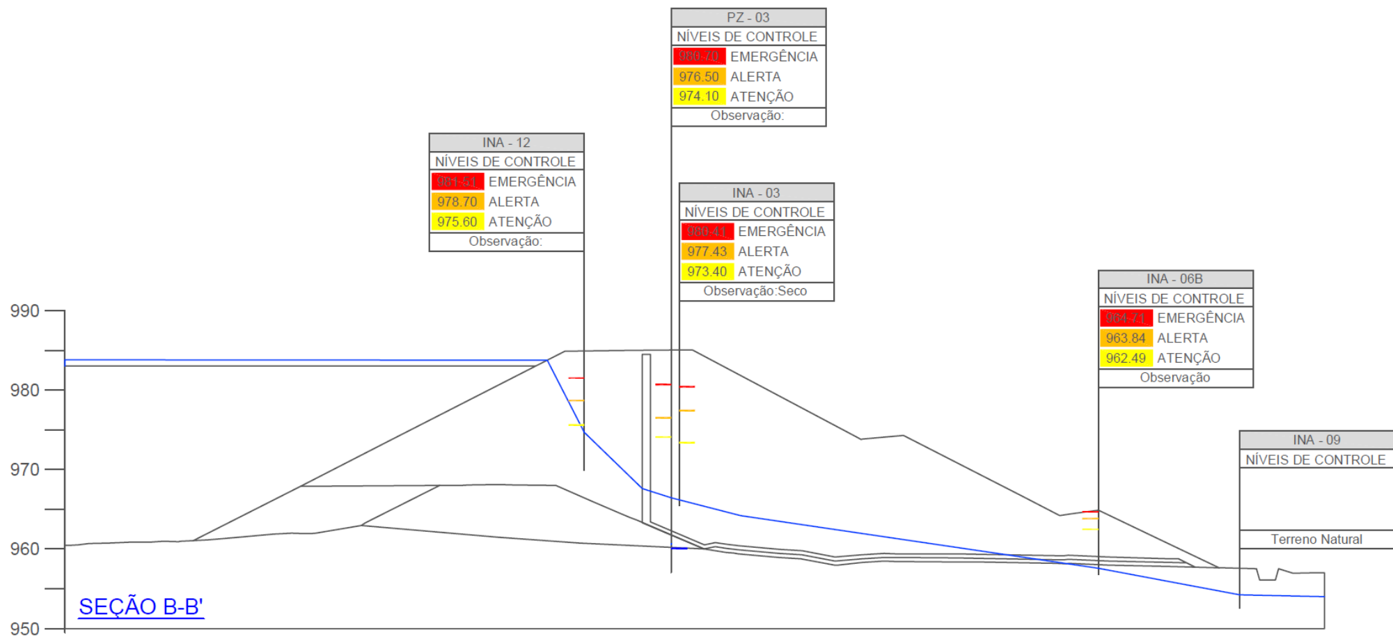
Figura 3 – Seção B-B'
