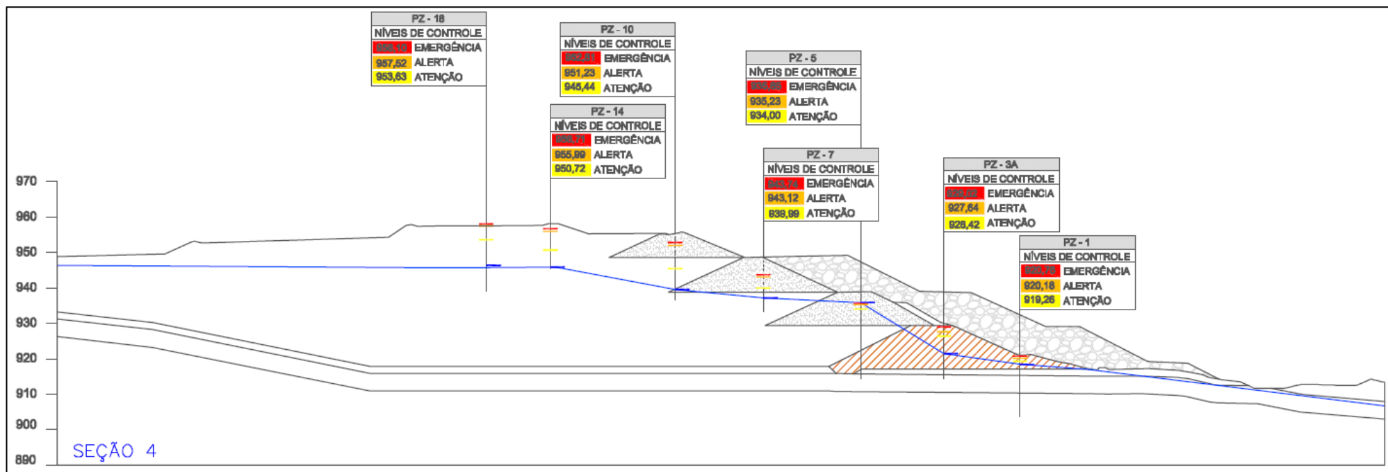
Figura 7 – Seção 04
