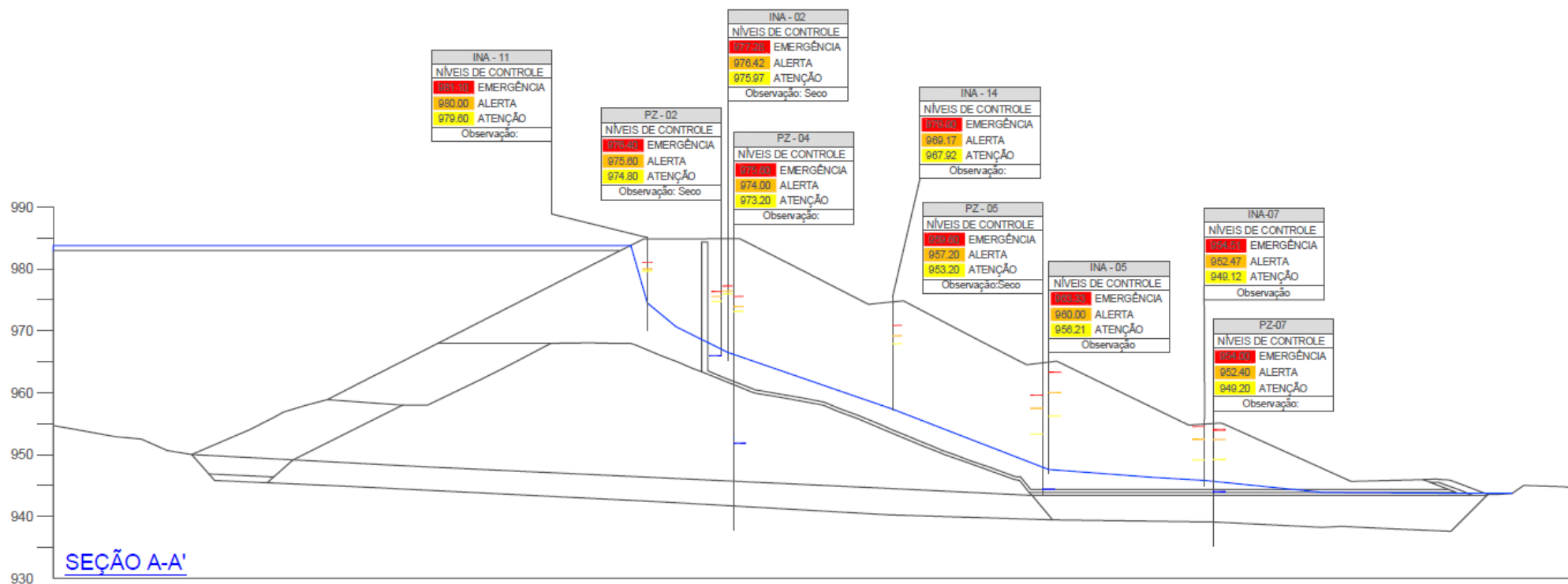
Figura 2 – Seção A-A'
