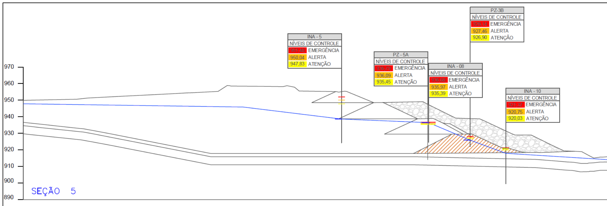
Figura 8 – Seção 05
