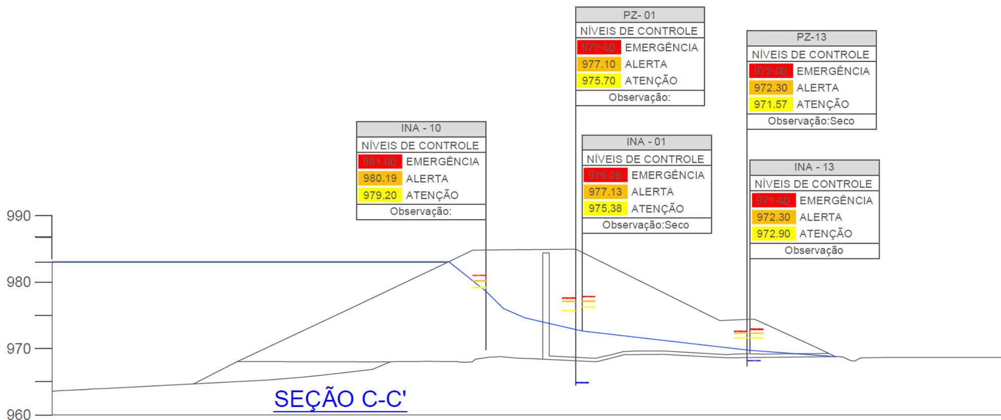
Figura 4 – Seção C-C'
