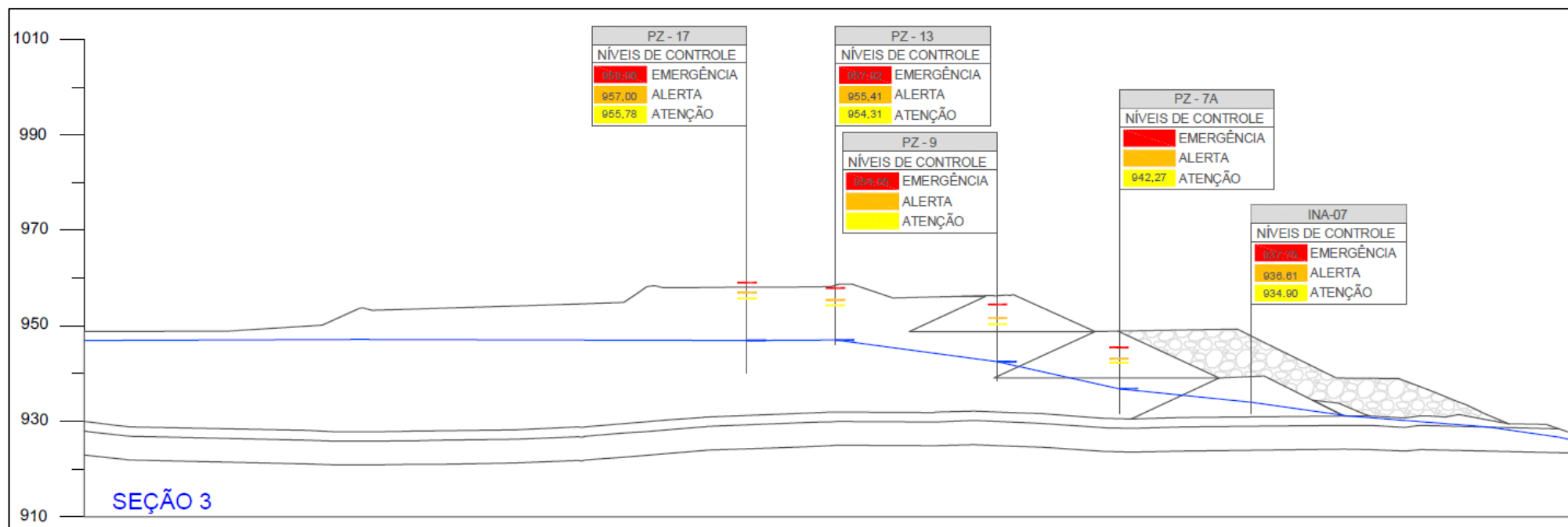
Figura 6 – Seção 03
