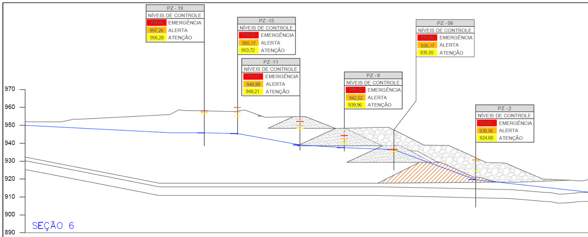
Figura 9 – Seção 06
